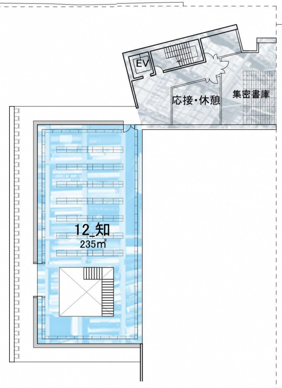
2F平面図 1/400
